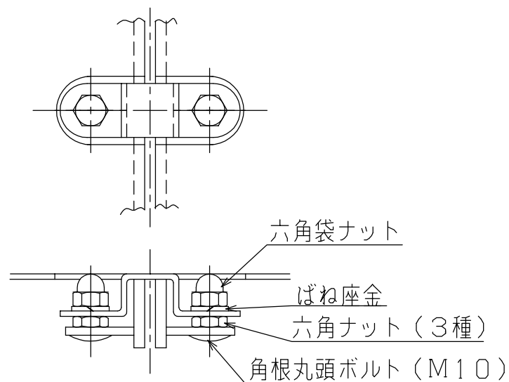
A部取付状態図 S = 1 / 3
