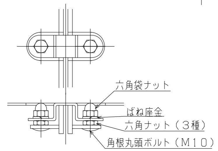
A部取付状態図 S = 1 / 3
