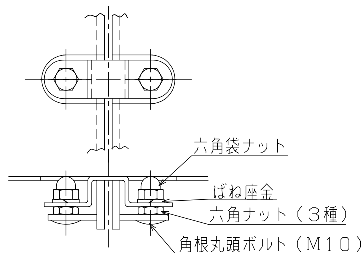
A部取付状態図 S = 1 / 3
