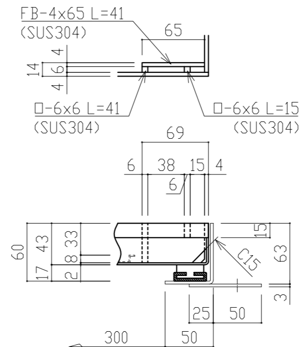
【 把手穴部詳細図 】 S:1/4
