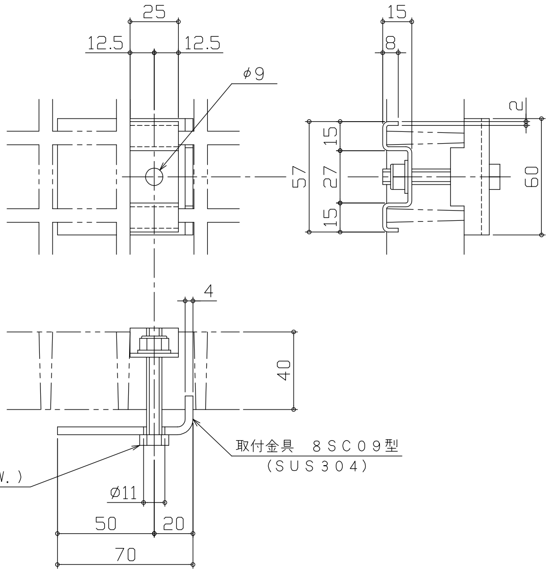
取付金具詳細 S = 1 / 2 8SC09型
