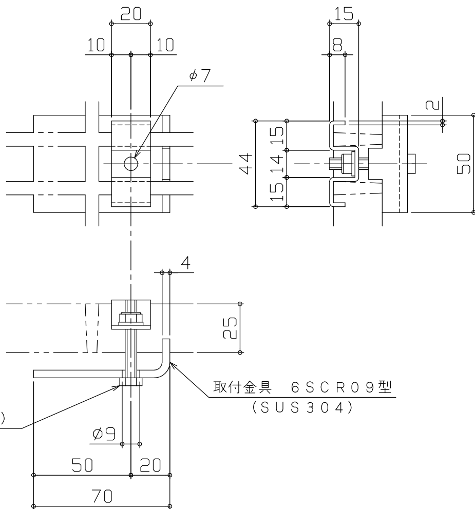
取付金具詳細 S = 1 / 2 6SCR09型
