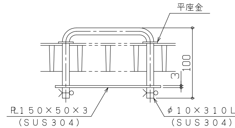
取手詳細
