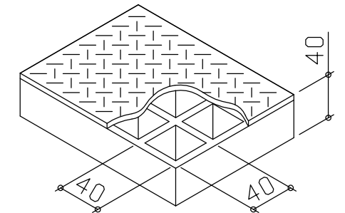
板貼仕様FRPグレーチング詳細
