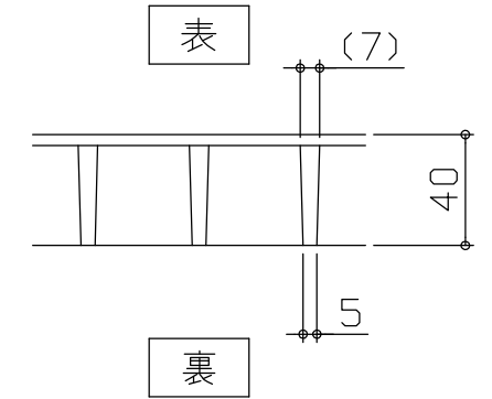
FRPグレーチング断面図 (板貼仕様)
